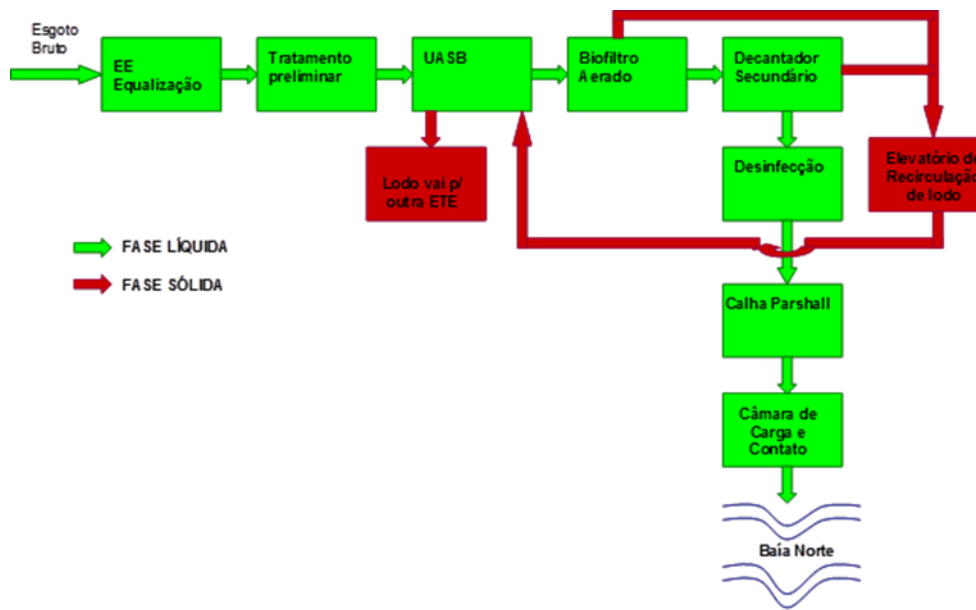
Figura 2: Fluxograma da ETE Saco Grande
